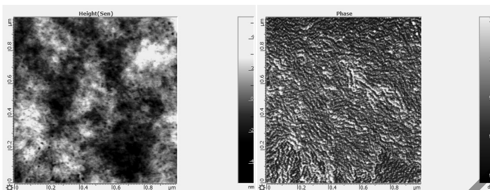
Рисунок 2. Фотоактивная пленка РЗНТ:РСВМ. Рельеф поверхности и фазовый контраст, измеренные АСМ, до деградации
