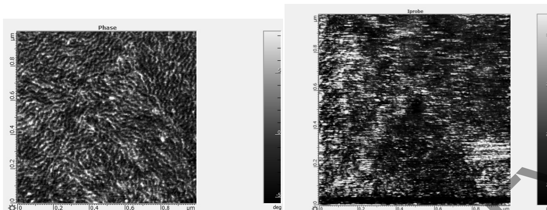
Рисунок 4. Распределения тока, измеренные АСМ на поверхности пленки РЗНТ:РСВМ до (справа) и после облучения УФ (слева)
