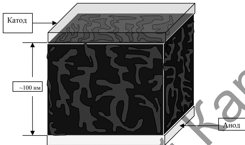
Рисунок 1. Схема ОСЯ на основе объемного гетероперехода
