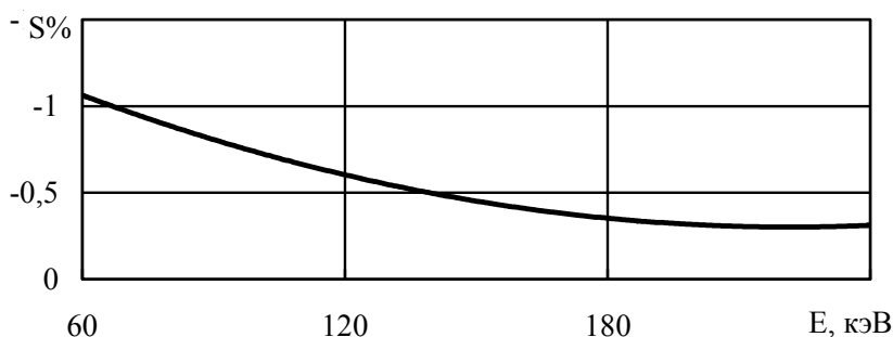
Рис. 4. Зависимость чувствительности метода ГТК-С к содержанию железа от энергии гамма-излучения
