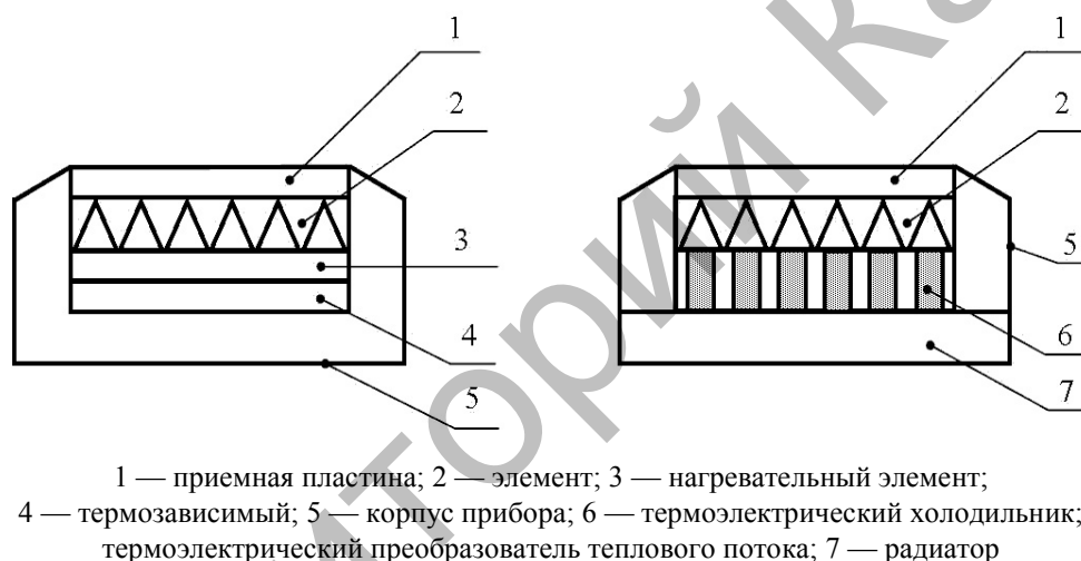
Рисунок. Схематическое изображение измерителя теплового потока
