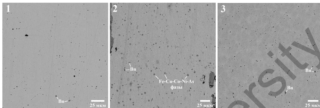
Рис. 3. Минеральные включения в металлических изделиях:
