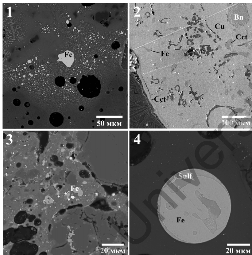
Рис. 5. Включения железа в медных шлаках позднего бронзового века:
