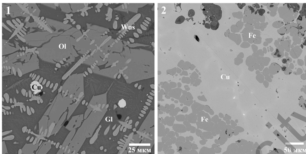
Рис. 4. Минералогия железосодержащих артефактов:
