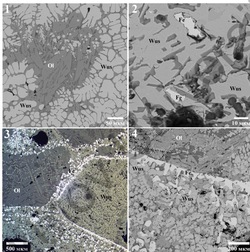
Рис. 6. Минералогия и текстурно-структурные особенности железных шлаков:
