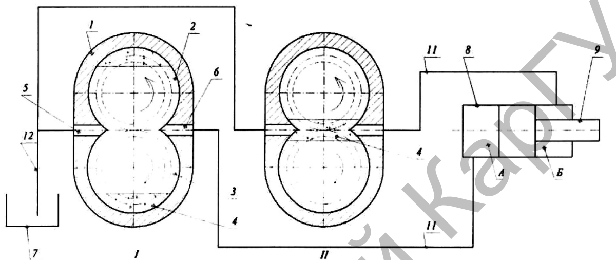
Рисунок 4. Спаренный насос шестеренный импульсный
