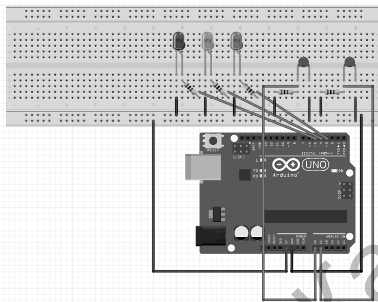
Рисунок 7. Схема подключения для работы программы Arduino&LabVIEW в макетной плате
