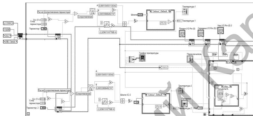
Рисунок 9. Блок-схема программы
