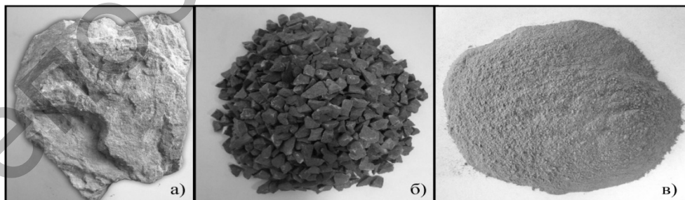
а — металқұрамды шикізаттың фотосуреті; б — механикалық бөлшектегіштер мен ұнтақтағыштарда өңделген өнім; в — электроимпульсті технологияда өңделген шикізаттың ұнтағы
