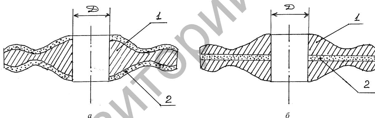
а — упрочнение приповерхностных слоёв; б — упрочнение серединной части
