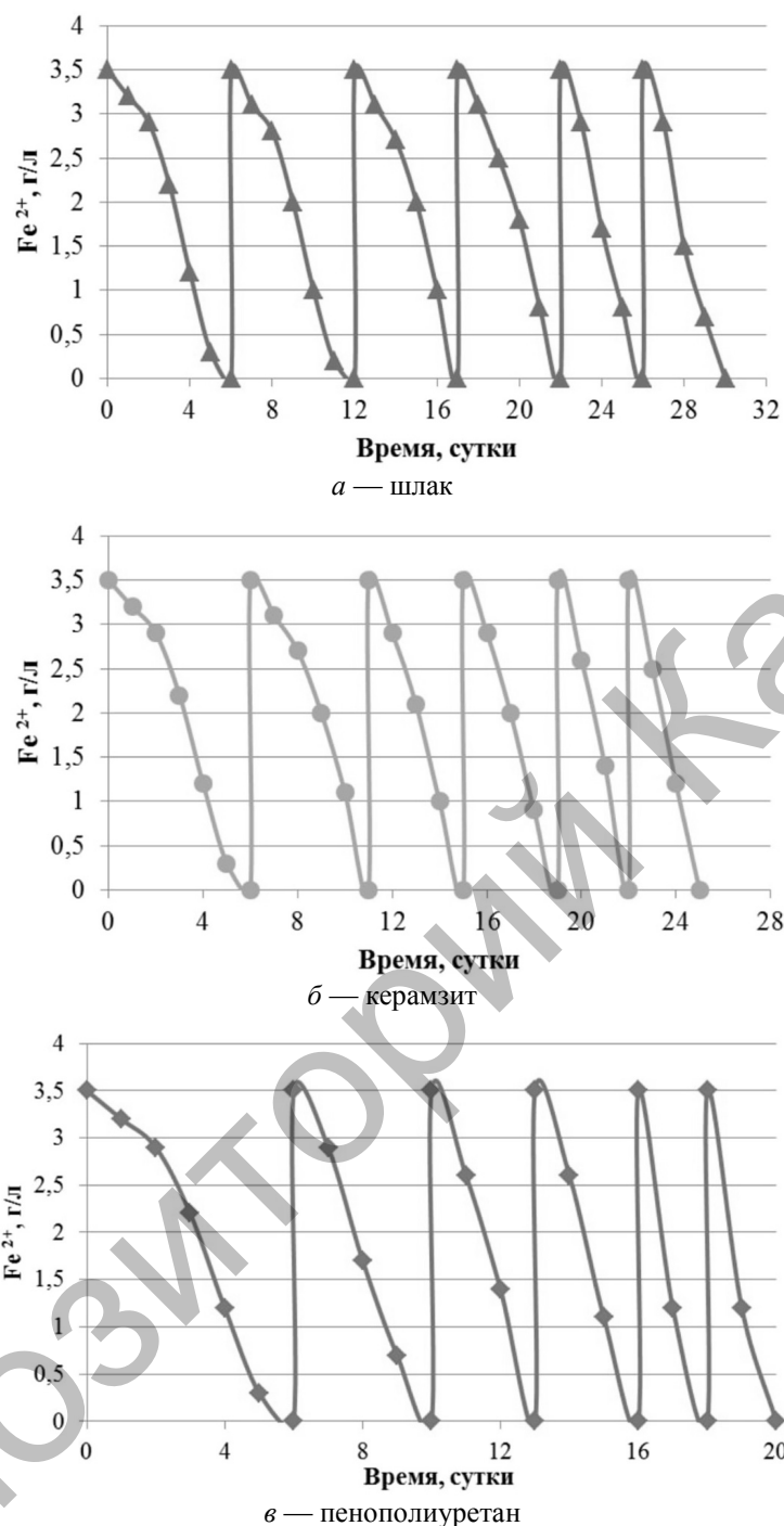
Рисунок 1. Динамика окисления \text{Fe}^{2+} при последовательном многоступенчатом культивировании консорциума микроорганизмов, иммобилизованного на инертных носителях
