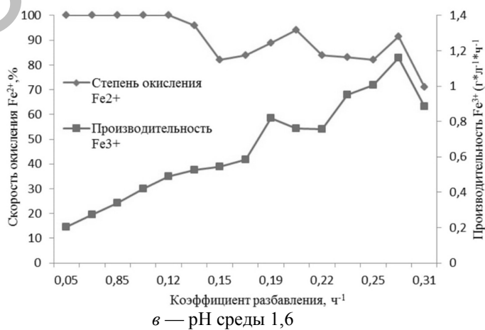
Рисунок 2. Производительность трехвалентного железа и степень окисления двухвалентного железа в проточном биореакторе, иммобилизованном бактериями, при различных концентрациях серной кислоты
