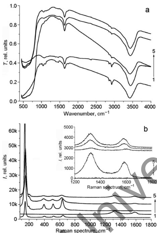
Fig. 2. IR (a) and Raman spectra (b) of samples: 1) TiO 2 , 2) rGO, 3) TiO 2 -rGO/1%, 4) TiO 2 -rGO/5%, and 5) TiO 2 -rGO/10%.
