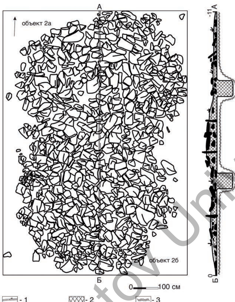
Рис. 2. Кетабан. План и профиль сооружения 2: 1 – дёрн; 2 – коричневый слой; 3 – материк 2-сур. Кетабан. 2-құрылыстың сызбасы мен профілі: 1 – қара топырақ; 2 – қоңыр топырақ; 3 – материк
