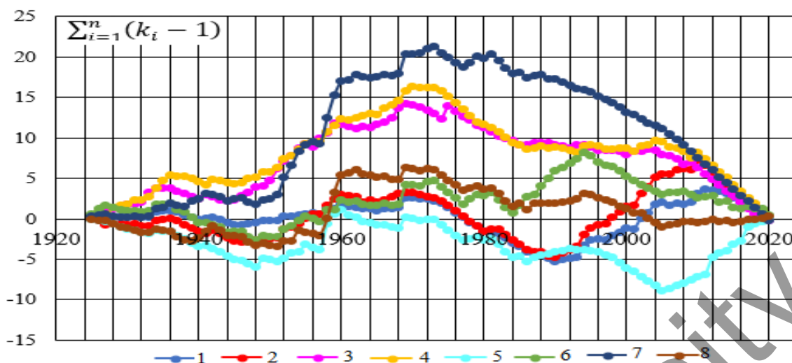
Рисунок 10. Разностно-интегральная кривая среднегодового расхода воды реки Куркюреу-Суу по гидрологическим постам Чон-Кургак (1) и Маймак (2), реки Терс (3), Асса (4), Тамды (5), Беркуты (6), Коктал (7) и Шабакты (8) за 1925–2020 гг. и оценки водности (репрезентивности)
