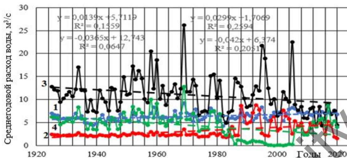
Рисунок 3. График изменения среднегодового расхода воды реки Куркуреу–Суу в гидрологических постах Чон–Кургак (1), Маймак (2), реки Ассы в гидрологическом посту Маймак (3) и реки Тер в гидрологическом посту Нурлыкент (4) за 1925–2020 годы и его линейный тренд
